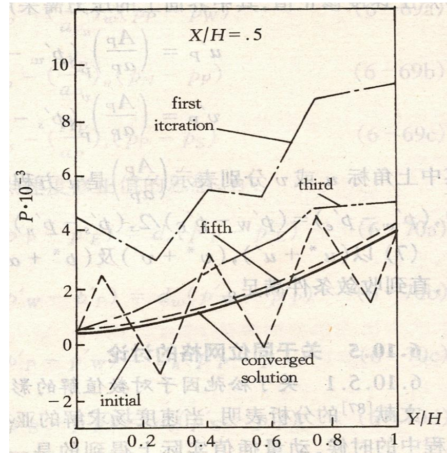
同位网格有效性的数值验证举例
