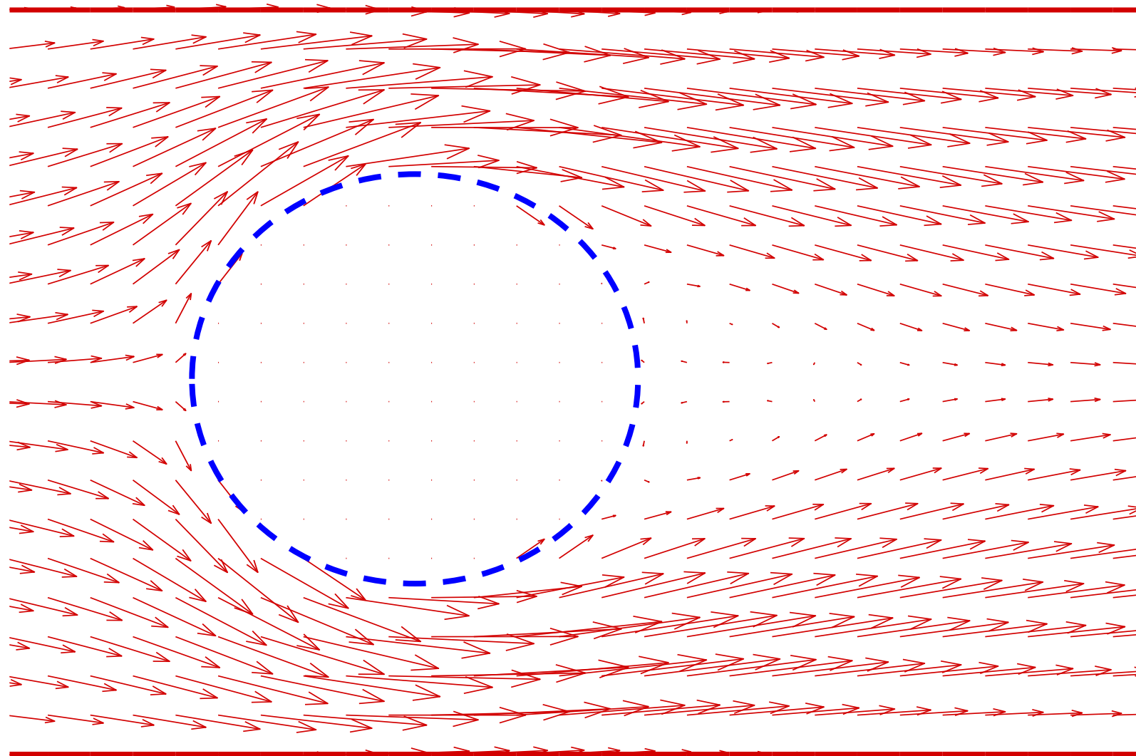
网格202X22 Re=100, 单元切割法
