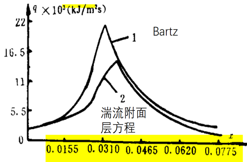
图 1 对流传热沿喷管长度的分布 ( t = 0.2s )
