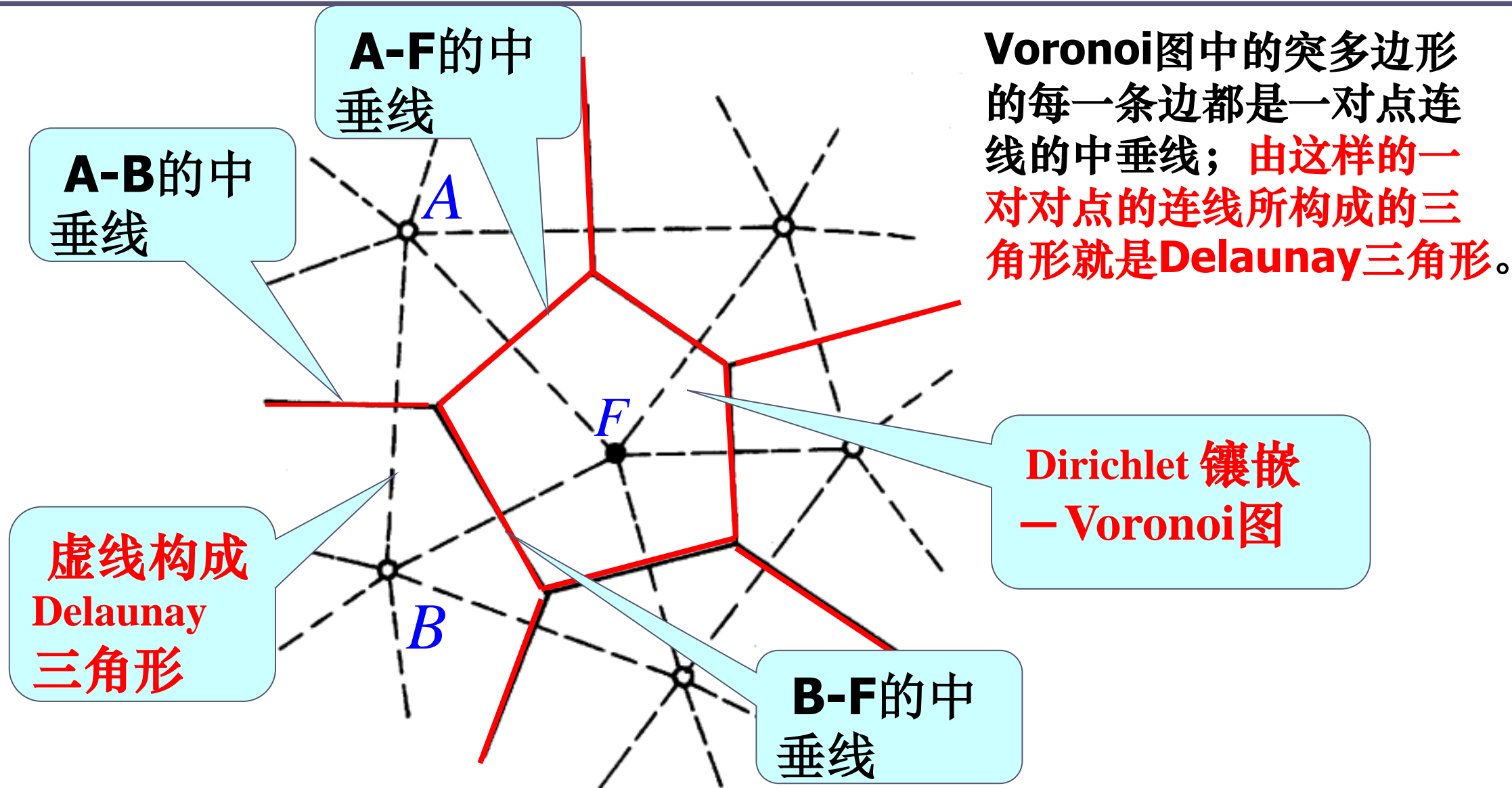
Dirichlet 镶嵌与Delaunay三角形的关系
