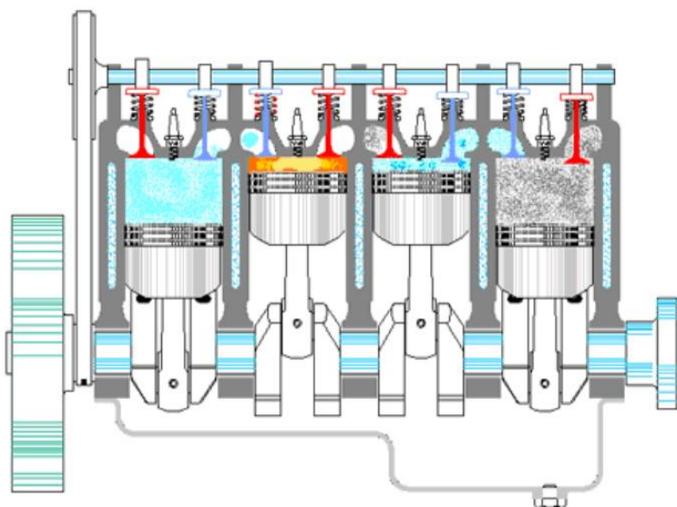
气缸中气体运动空间
