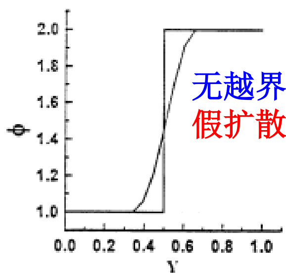
(f) OSHER (BDBD)
