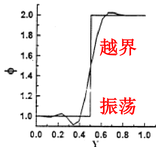
(d) QUICK 格式与精确解的比较
