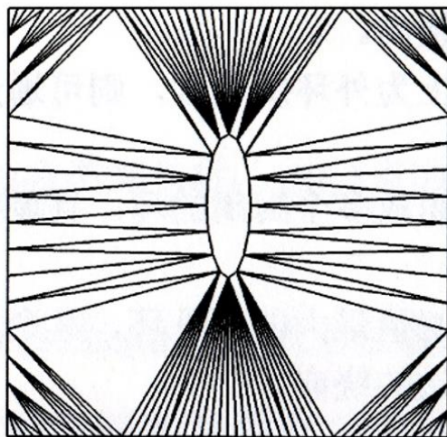
(b)映射到平面上用Delaunay方法生成初始网格
