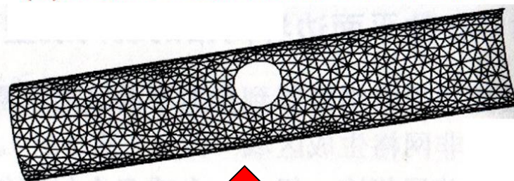
(d)映射到空间后的曲面网格
